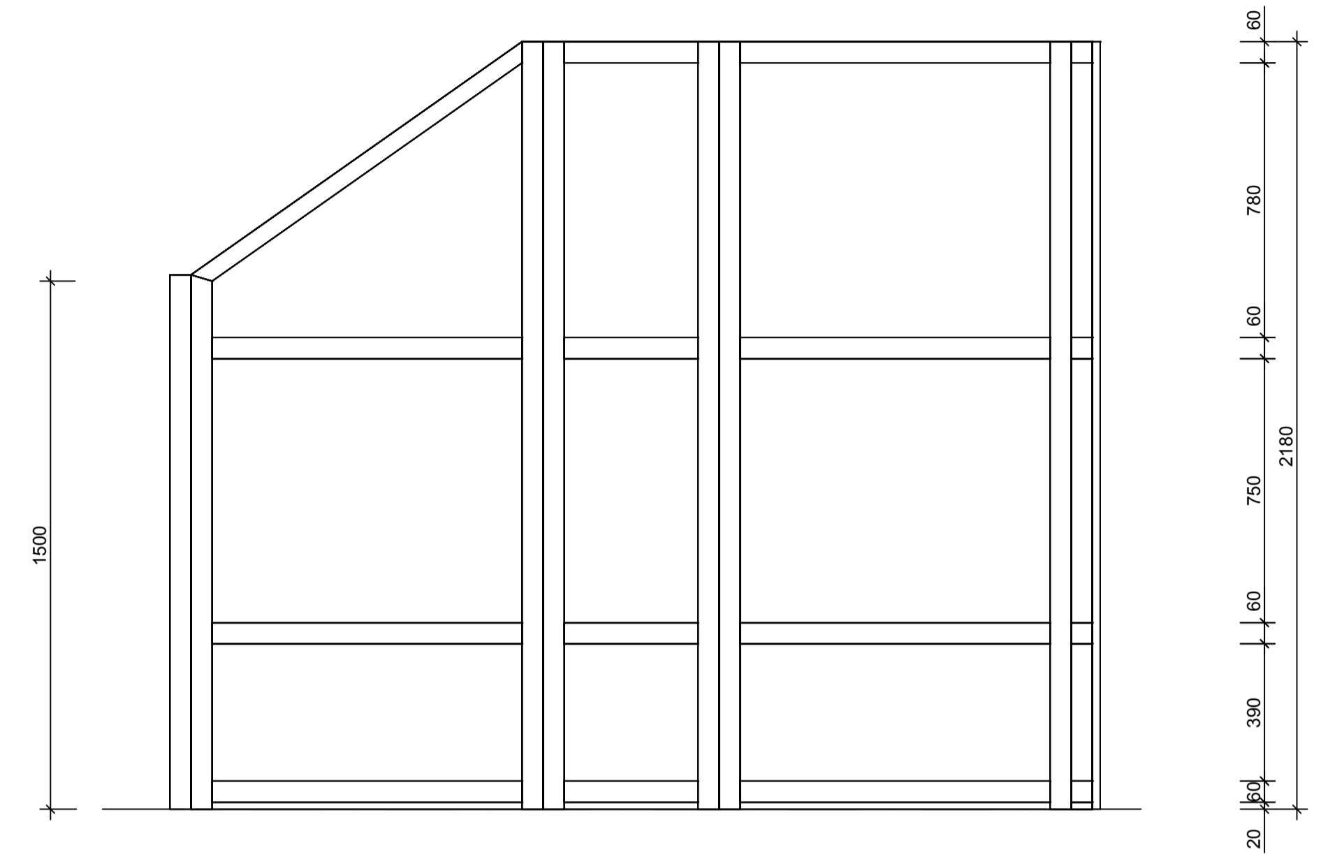
Ansicht Seitenwand links M 1:15
