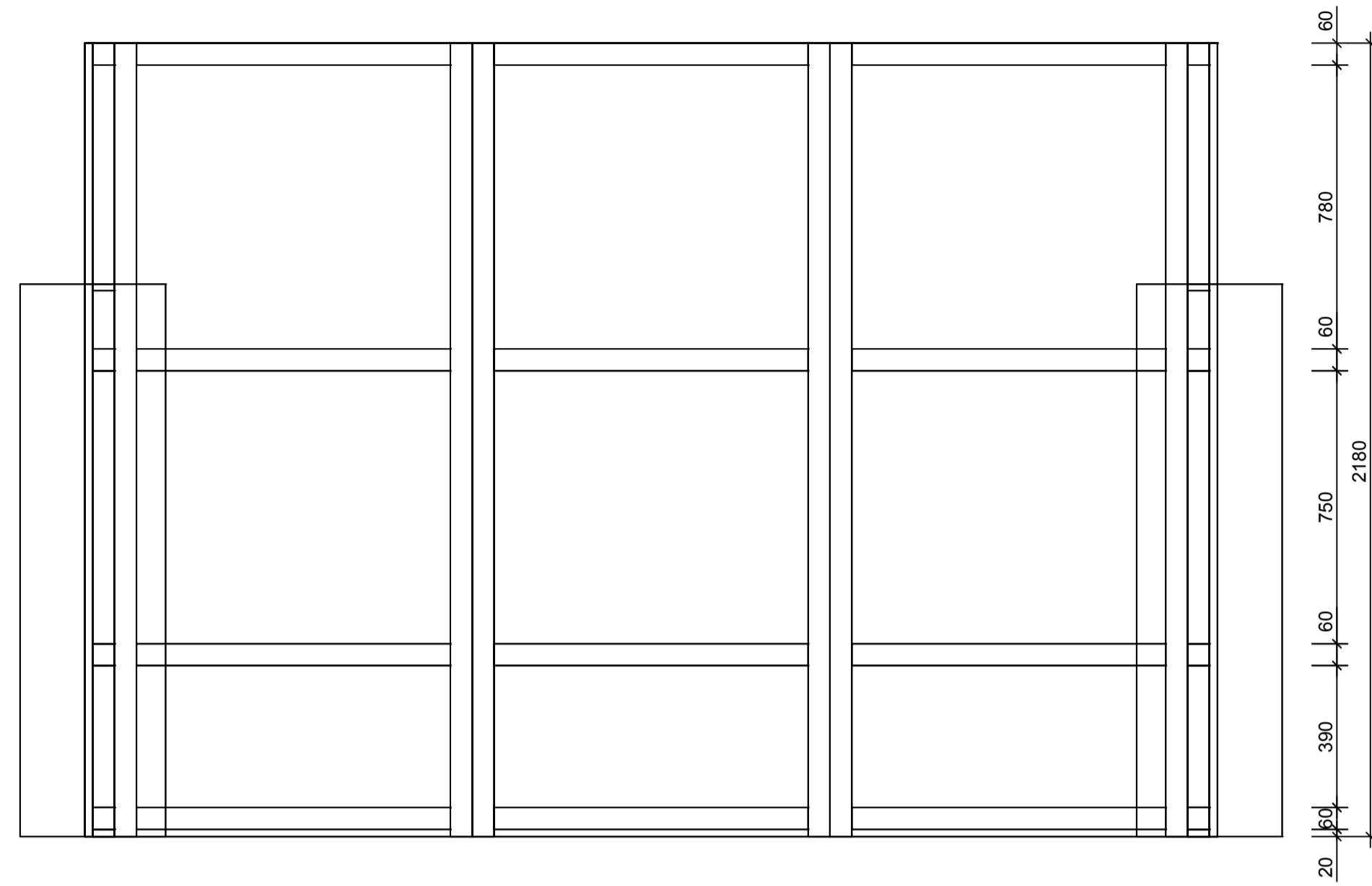
Ansicht Rückwand M 1:15
